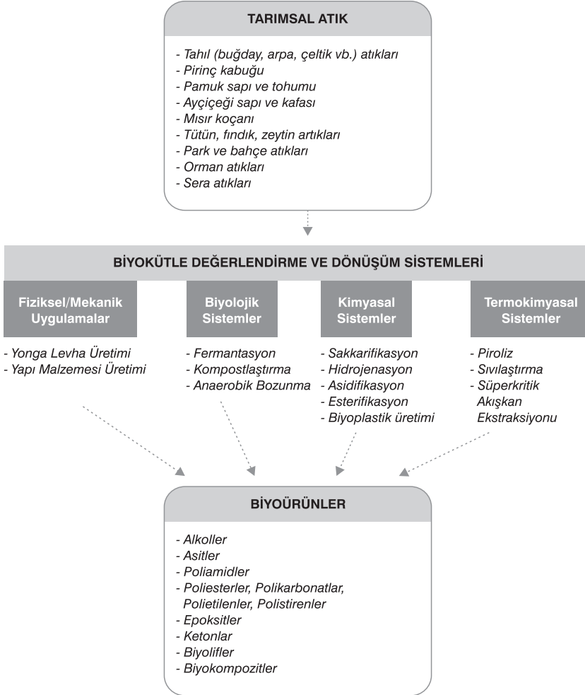
Şekil 1.1. Biyokütle Değerlendirme ve Dönüşüm Sistemleri (Yakıt Dışı)
